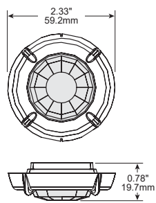
FSP-L2 dimensions
