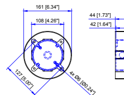
SCBT Surface Conduit Box Trim
