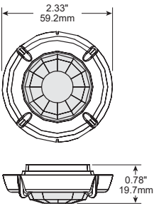
FSP-L2 dimensions
