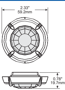
FSP-L2 dimensions
