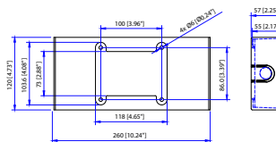
SCBT Surface Conduit Box Trim
